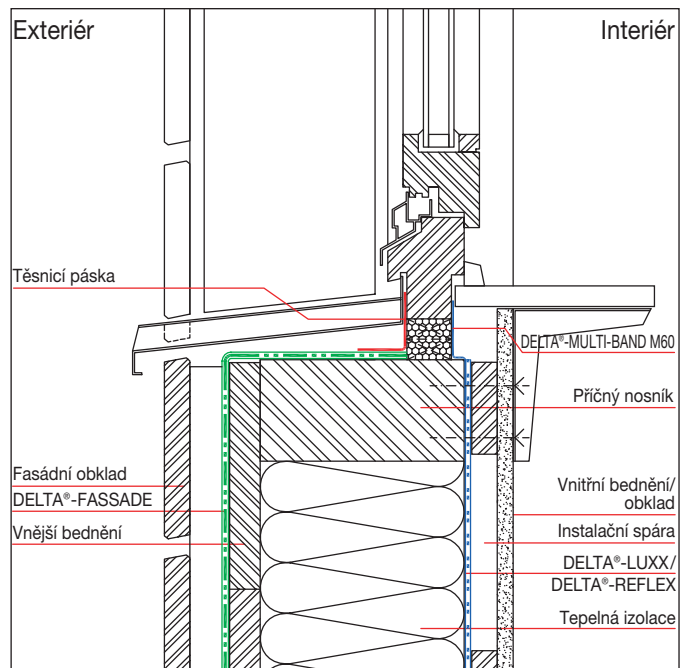
Napojení na okno – svislý řez, parapet
