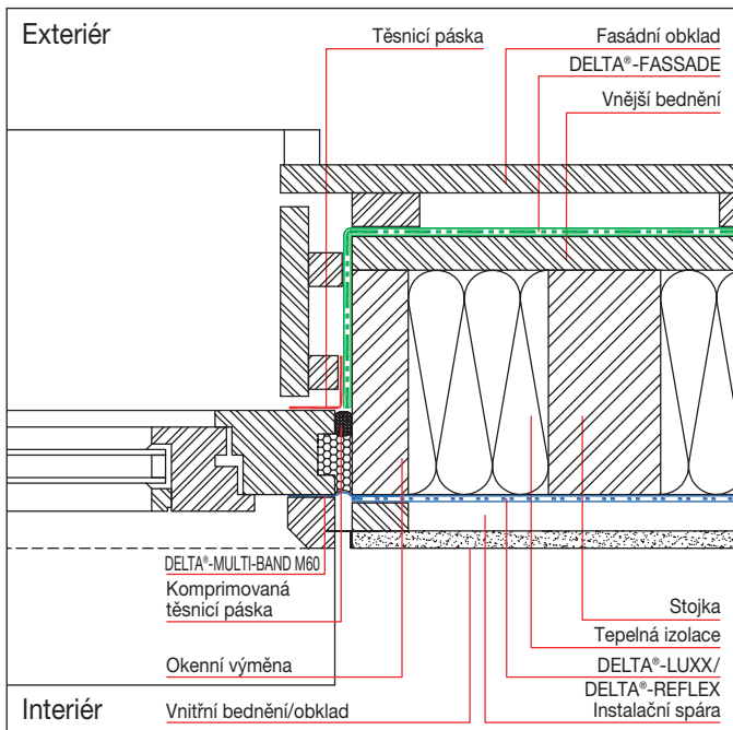
Napojení na okno – vodorovný řez
