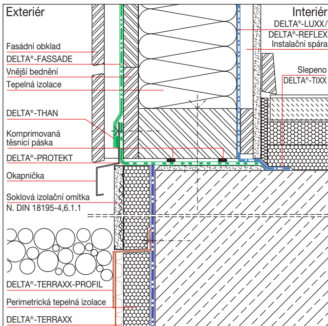
Přechod na základ
