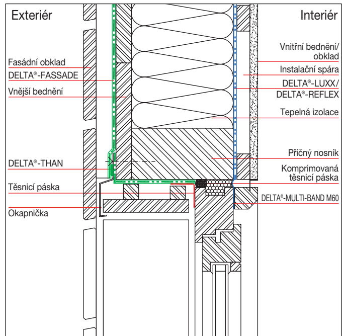
Napojení na okno – svislý řez, nadpraží
