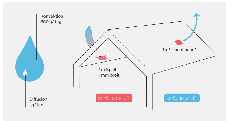
Im Vergleich zu den Feuchtigkeitsmengen, die über Diffusion in den Dachaufbau eindringen können, sind die Feuchtigkeitsmengen bei der Konvektion beträchtlich.
